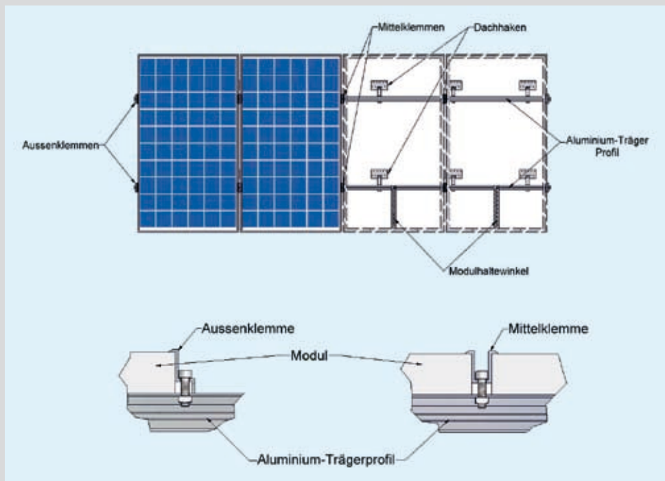
Aufbau Schrägdachhalterung
