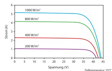
Strom-Spannungskennlinie bei verschiedenen Einstrahlungswerten
