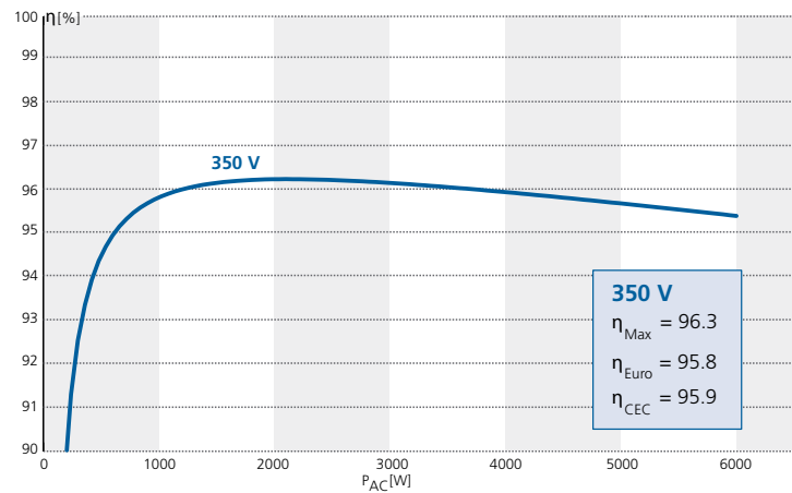
Wirkungsgradkennlinie Powador 6600
